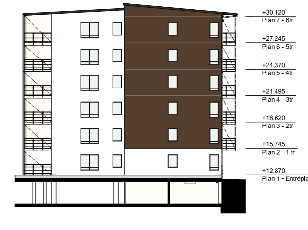
F3_V Tr 3, Gärdsfasad mot väster 1:200
