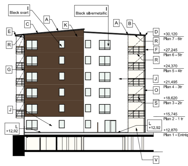
F2_Ö Tr 2, Gärdsfasad mot öster 1:200
